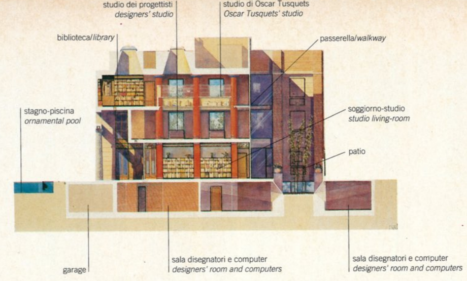
sezione longitudinale sullo stagno-piscina/longitudinal section of the ornamental pool
