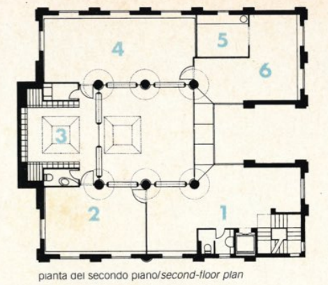
pianta del secondo piano/second-floor plan
