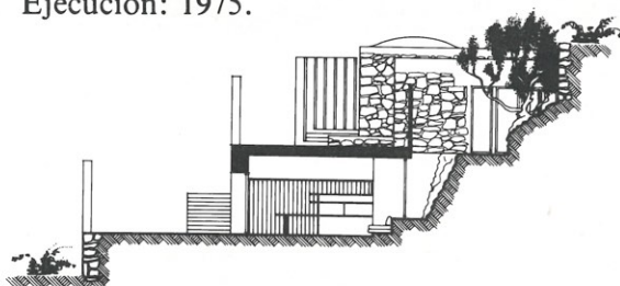
Sección transversal.
