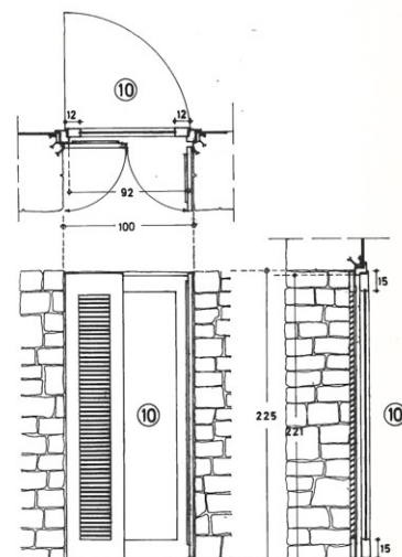
5 y 10: Detalles de carpintería. Cerramiento al interior y al exterior. 6 y 7: Carpintería interior.
